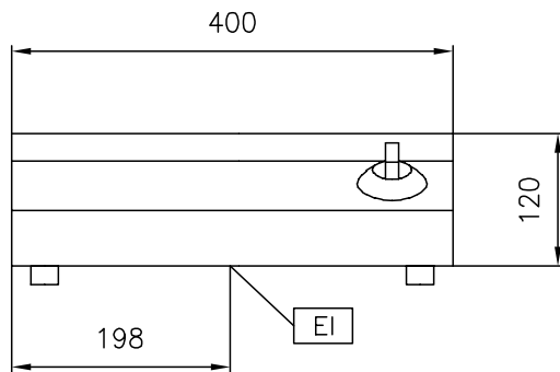
Front aanzicht
